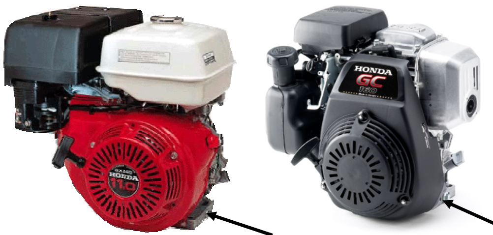
Рис. 4.7: Удаление винта для слива масла
