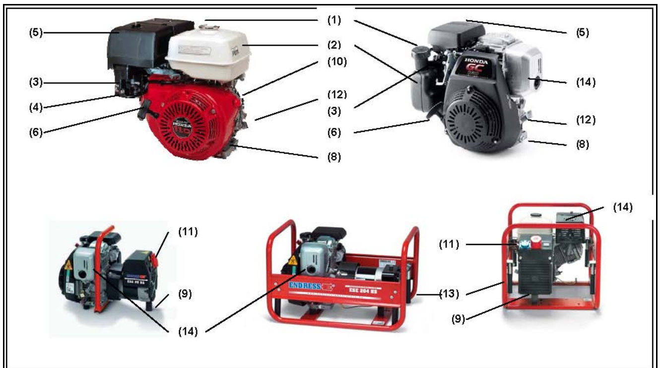
Рис 3.1. Элементы электростанции
