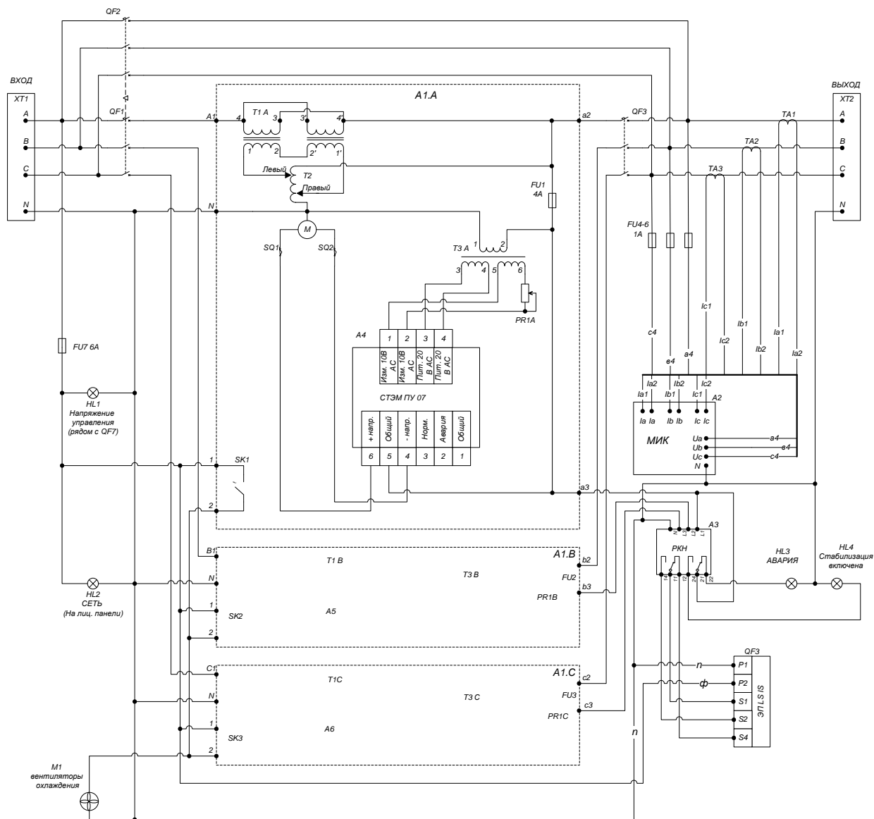
Рисунок 2. Схема стабилизатора.
