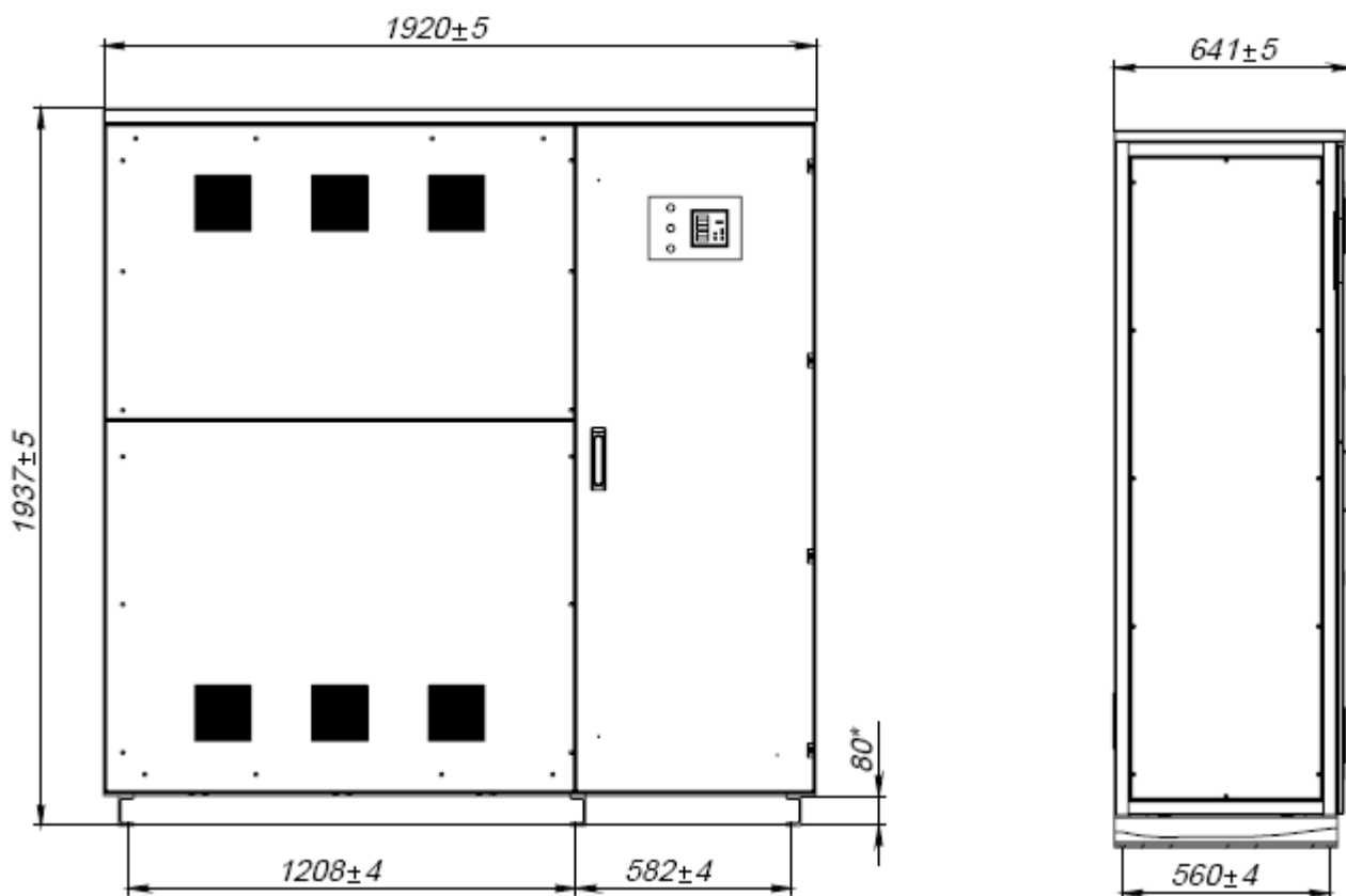
Рисунок 1. Габаритные размеры стабилизатора.
