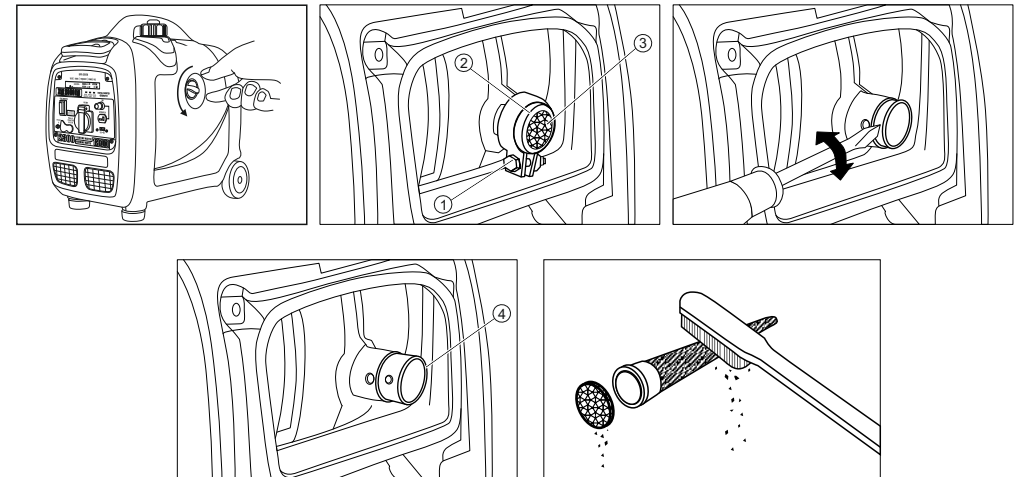
Рисунок 11 – Искрогаситель
