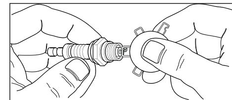
Рисунок 9 – Установка свечи
