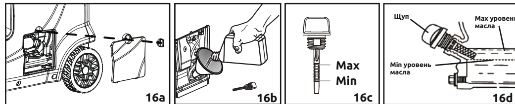
Рисунок 16 - Уровень масла
